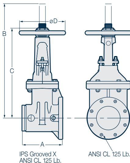
FLANGE X GROOVE FIG. 5093
