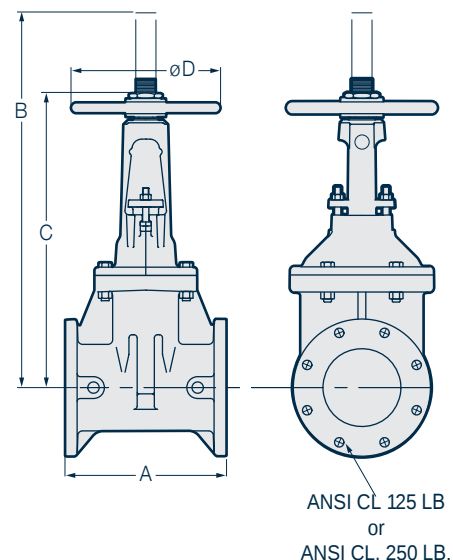
FLANGE X FLANGE FIG. 5068, 5168
